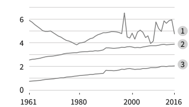
GtCO 2 Äq pro Jahr
